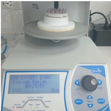
Imagen 6. Proceso de sinterización en laboratorio
